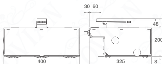
Rozměry pohonů BM4000/BM4024
