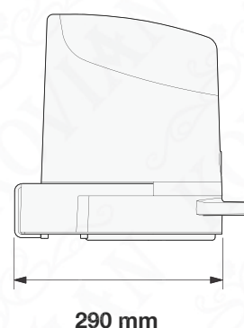
Rozměry pohonů HK7024/HK7224
