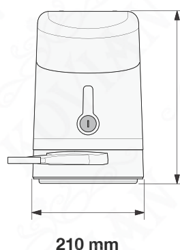
Rozměry pohonů HK7024/HK7224
