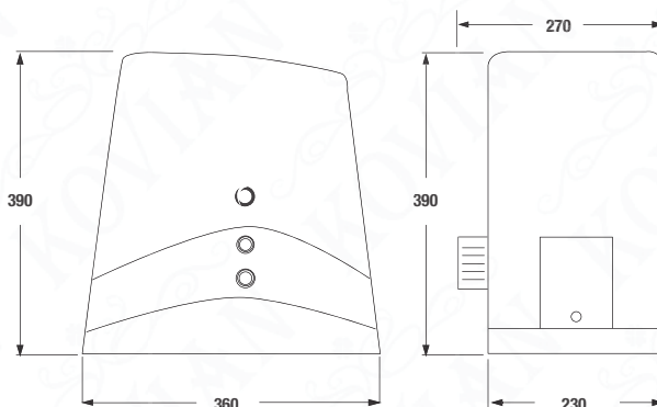
Rozměry pohonu TURBO200
