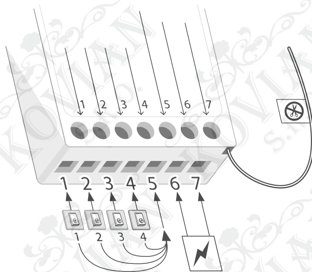
1 zapojení modulu
