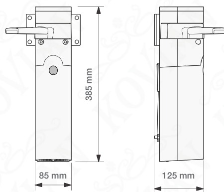
Rozměry pohonů WL1024C/WL1024
