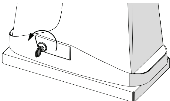
Fig. 8 IT - Sblocco di emergenza EN - Emergency unblocking FR - Déverrouillage d'urgence ES - Desbloqueo de emergencia
