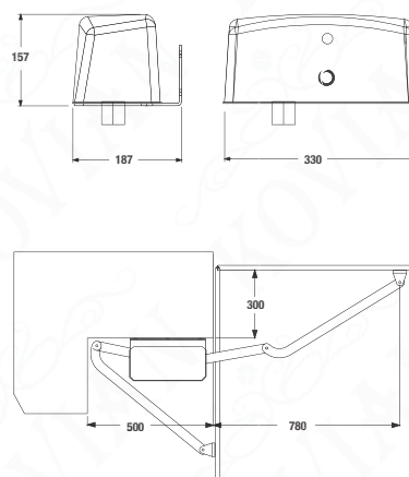
Rozměry pohonu MEWA
